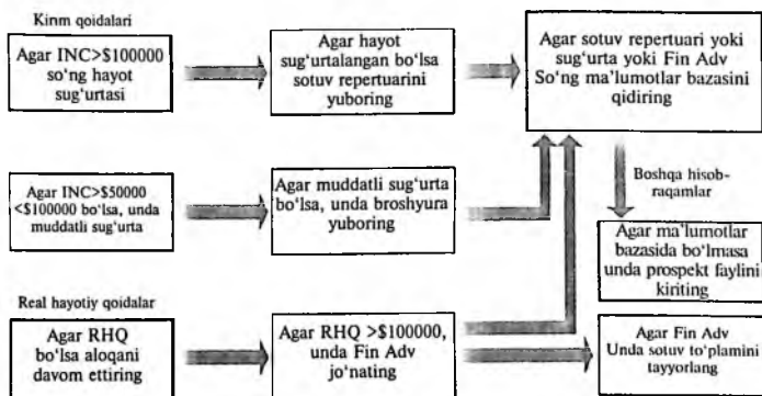
3.9.6-rasm. Ekspert tizimlaridagi mashinalar
