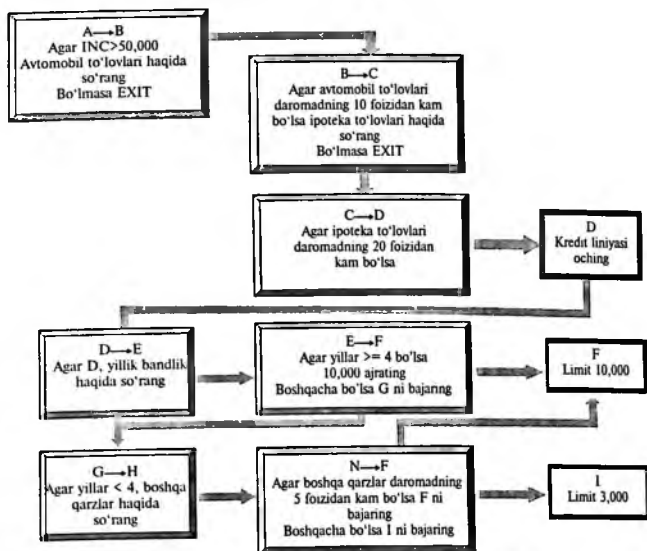
3.9.5-rasm. Ekspert tizimi qoidalari
