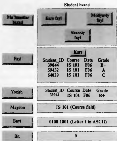
1.8.1-rasm. Ierarxik ma'lumotlar bazasi
