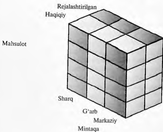
1.8.8-rasm. Ko'p o'lchamli ma'lumotlar modeli
