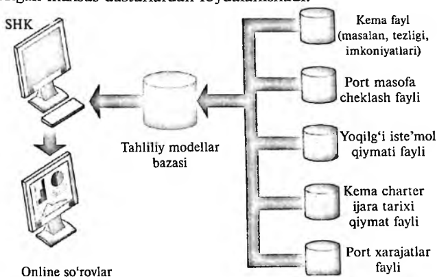
3.2.5-rasm. Voyage-baholash qaror qabul qilishni qo'llab-quvvatlash tizimi
