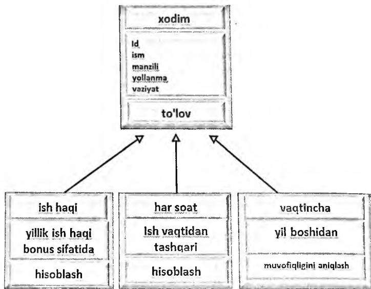
2.3.7-rasm. Tuzilma harakat sxemasi.
