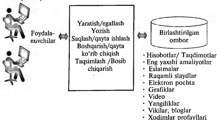
3.9.3-rasm. Korxona ichidagi boshqaruv tizimi
