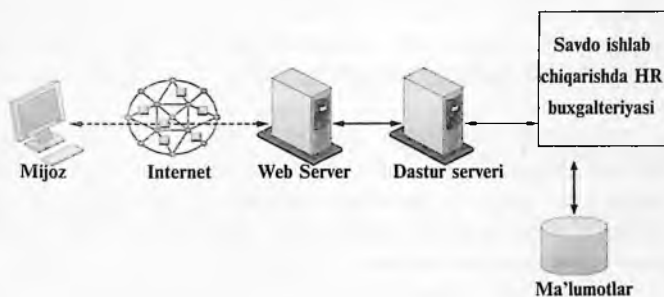
1.5.2-rasm. N-bosqichli bir necha qatlamli mijoz/server tarmog'i
