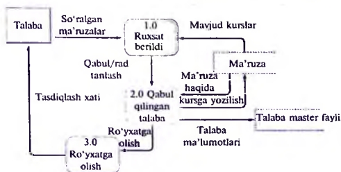
2.3.5-rasm. Ma'lumotlar oqimi diagrammasi
