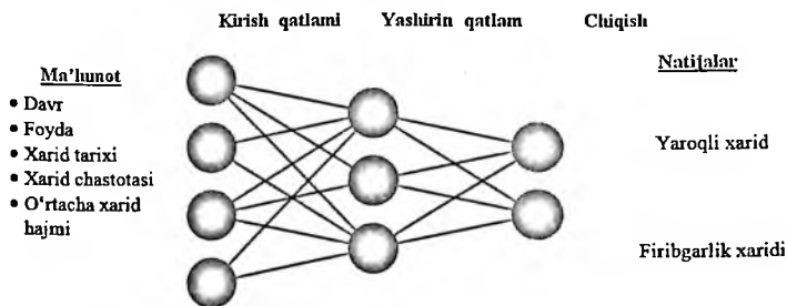
3.9.9-rasm. Neyron tarmog'i funksiyasi
