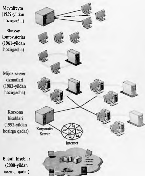
1.5.1-rasm. IT infratuzilmasining evolutsiyasi davrlari
